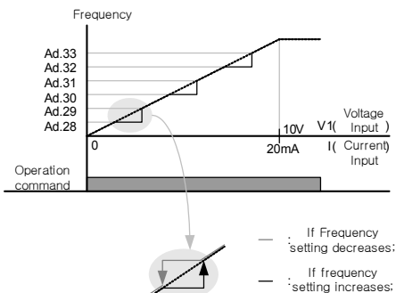
图 6-33 跳频曲线
