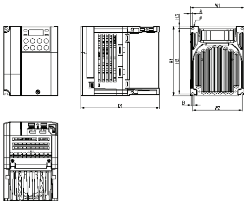
图 2-2 0008~0015S100(单相 200V), 0015S100~0022S100 (3 相 200V/400V)
