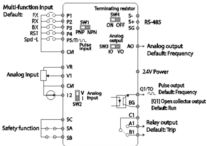
图 4-5 控制回路端子接线图
