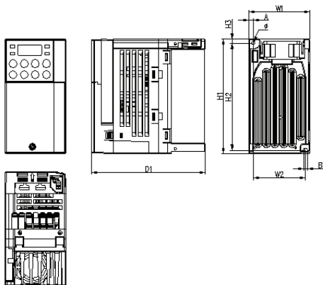
图 2-10004S100(单相 200V), 0004S100~0008S100 (3 相 200V/400V)
