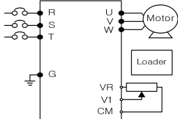
接线图
