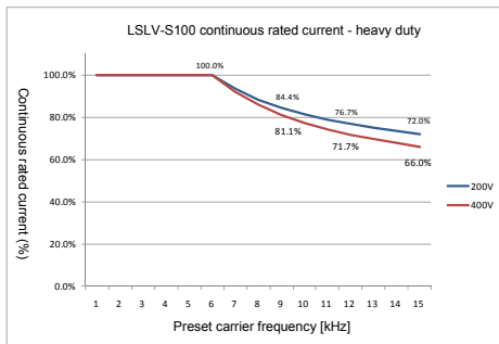
图 2-5 重载时连续额定电流
