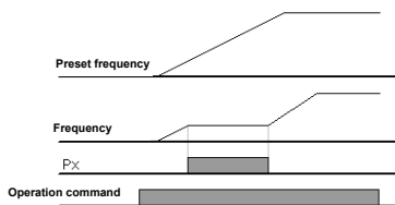
图 6-10 固定模拟量指令频率
