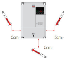
图 3-1 环境温度测量位置
