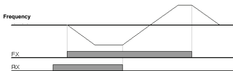
图 6-13 端子台运行指令 2
