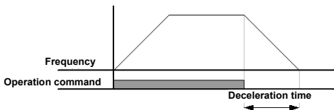
图 6-29 减速停止
