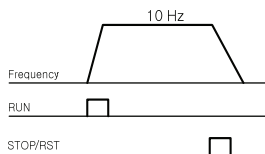
运行曲线
