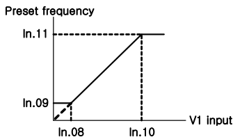
图 6-3In.08 V1 Volt x1 ~ In.11 V1 Perc y2
