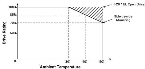
图 2-9 根据环境温度安装方法的连续额定电流
