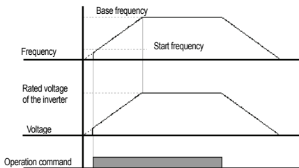
图 6-23 以起始频率以上运行的状态下减速停止时
