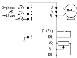
接线图
