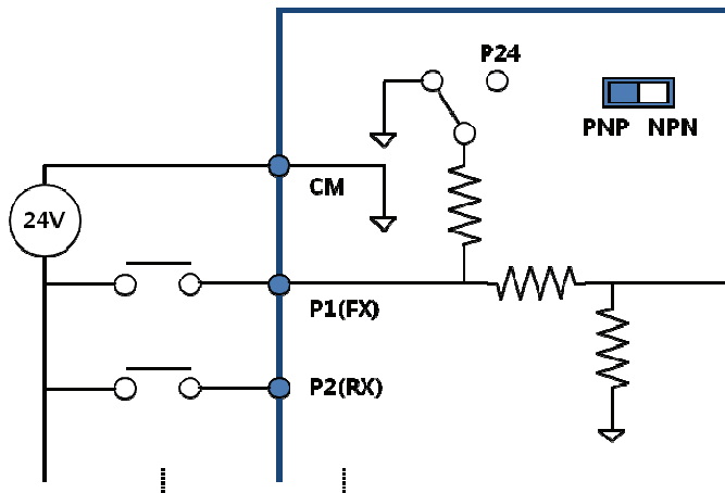
图 4-7 PNP 模式 (Source 模式)
