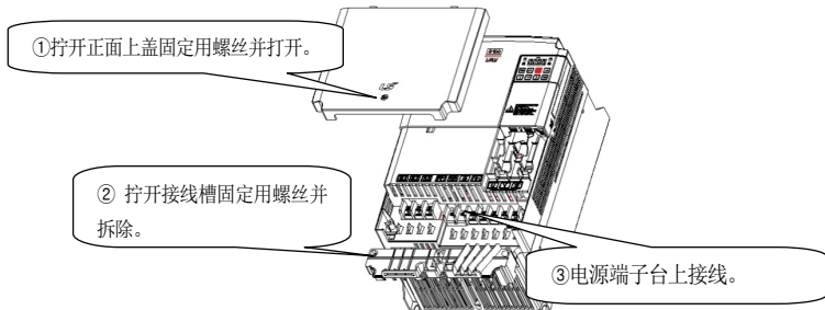
图 4-2 正面上盖级接线槽拆除方法(15kW 200V ~22kW 200/400V)
