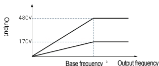
图 6-27 输入电源和电机电压规格不同时设置电机电压的情况
